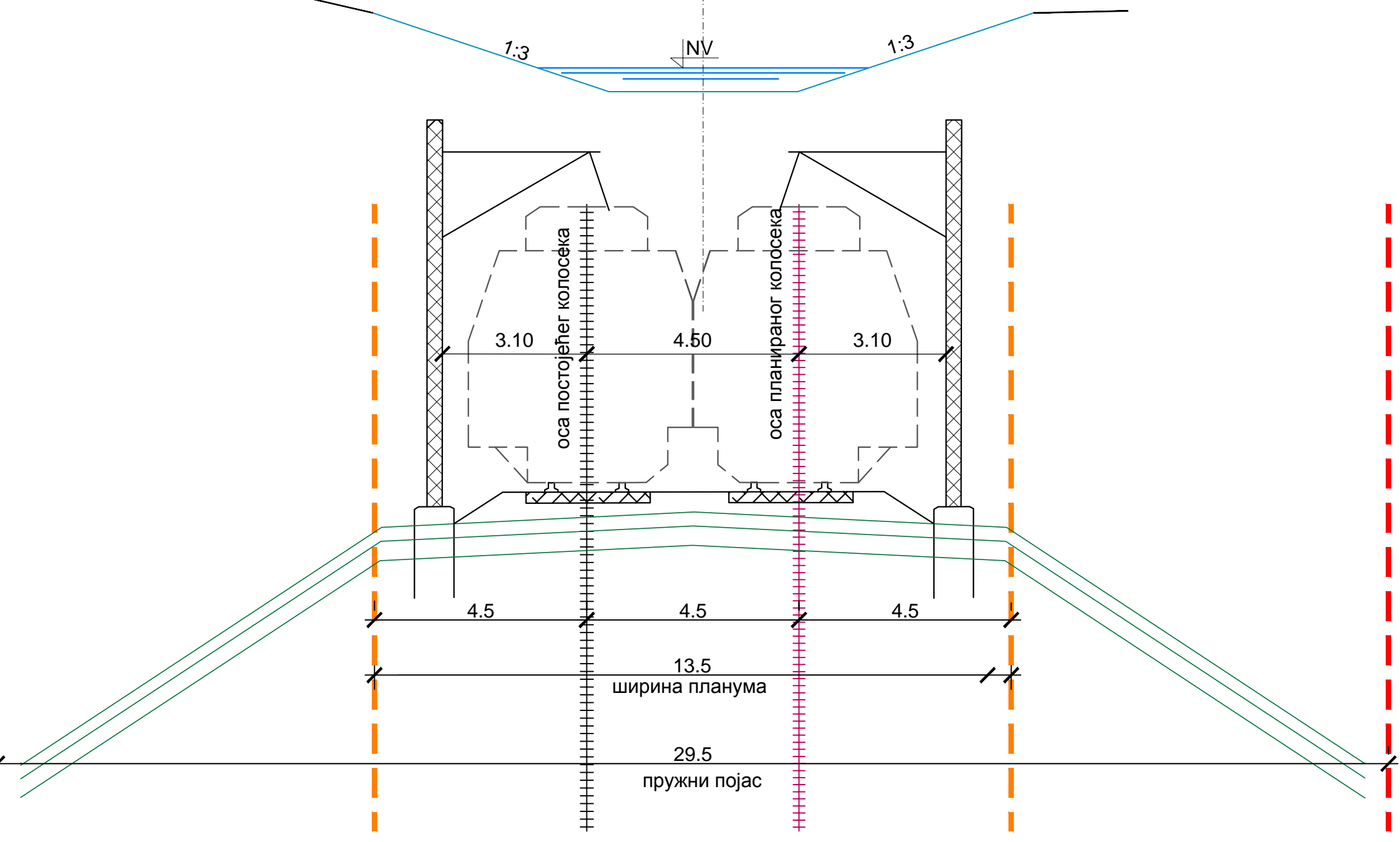
КАРАКТЕРИСТИЧНИ ПРОФИЛ БЕЛЈЕШЕВСКЕ РЕКЕ
