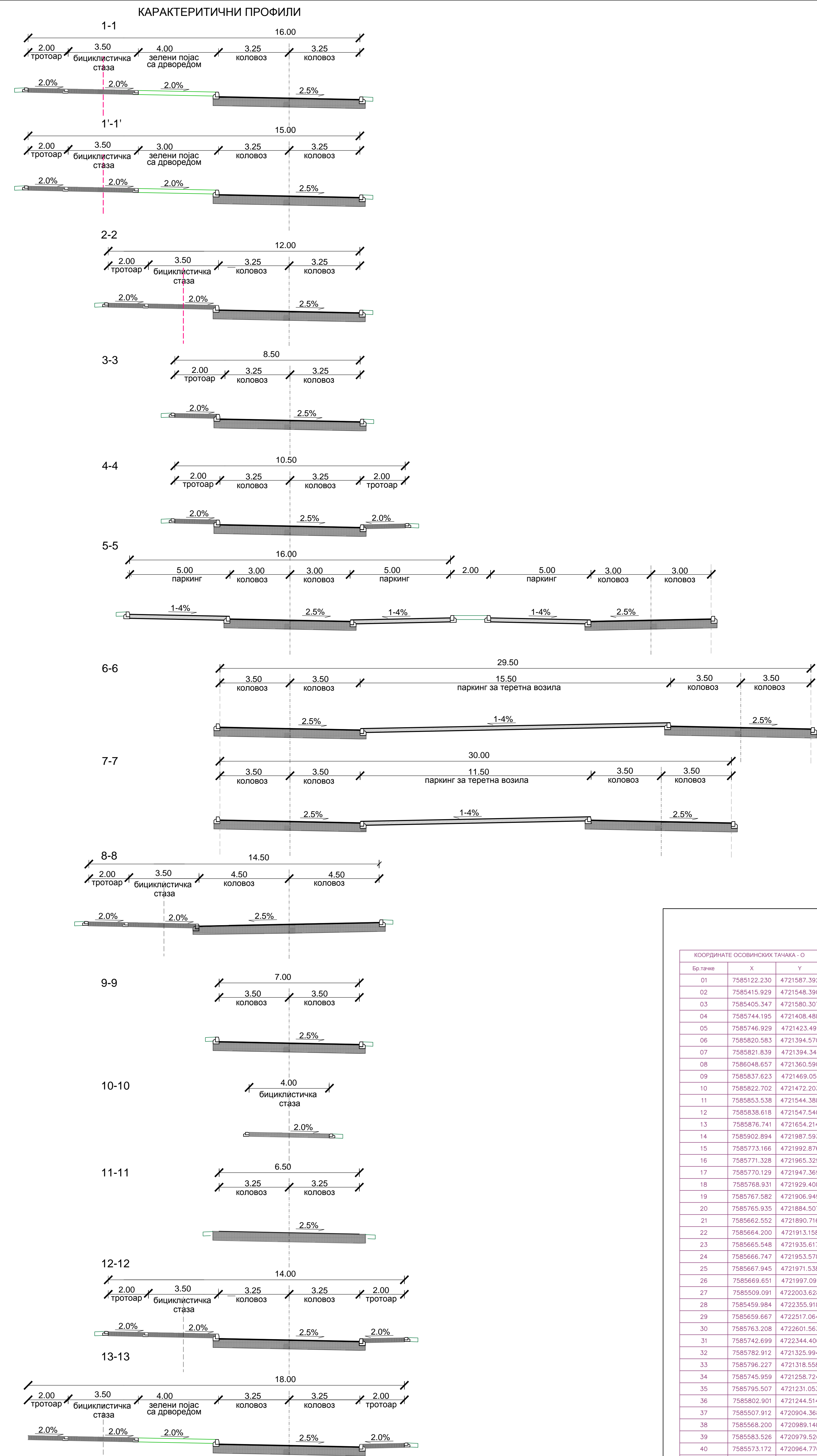
КАРАКТЕРИСТИЧНИ ПРОФИЛ БЕЛЈЕШЕВСКЕ РЕКЕ
